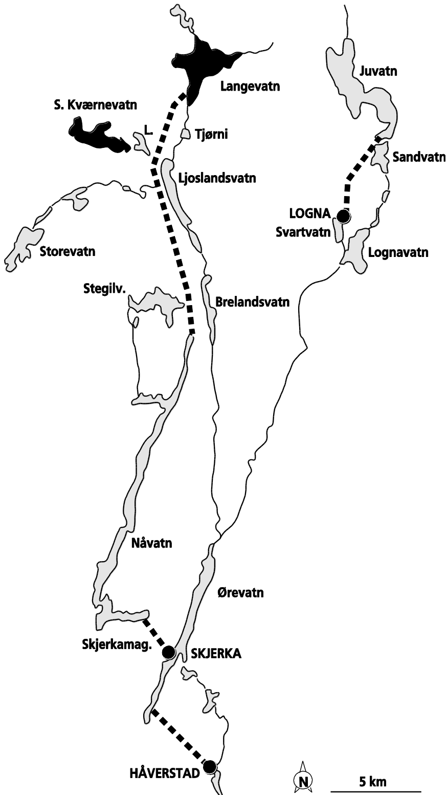
Figur 2. Kart over øvre deler av Mandalsvassdraget med overføringstuneller til og fra Nåvatn.
