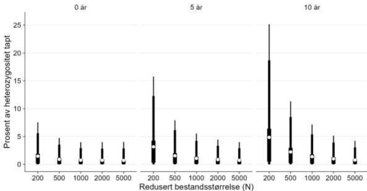
Figur 9: Tap av heterozygositet over 100 år, hvor en starter med bestandsreduksjon som holdes i 0, 5 eller 10 år. 90 % av voksen bukk høstes i perioden med redusert bestand og bestanden holdes stabil ved å skalere høstingsratene til kalv,
