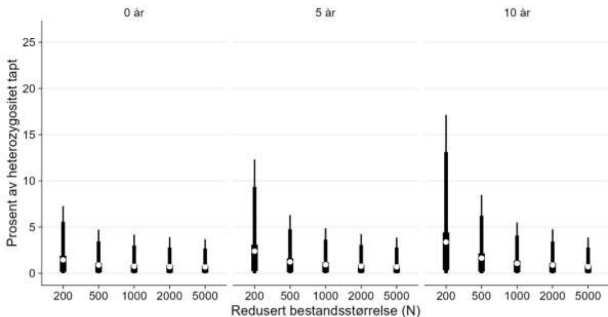
Figur 11: Tap av heterozygositet over 100 år, hvor en starter med bestandsreduksjon som holdes i 0, 5 eller 10 år. 50 % av kalvene høstes i perioden med redusert bestand og bestanden holdes stabil ved å skalere høstingsratene til ungdyr og voksen simle. Høstingsraten til voksen bukk holdes da ved gjennomsnittet i perioden 2005-2018 ( h_{m,2} = 0,156 ). N_0 = 7725 , p_0 = 0.5 og etter perioden med bestandsreduksjon opphører all høsting slik at bestanden vokser inntil den når N_0 . Ved N_0 holdes bestanden stabil ved å skalere alle de gjennomsnittlige høstingsratene. Skalerte høstingsrater tar som utgangspunkt
