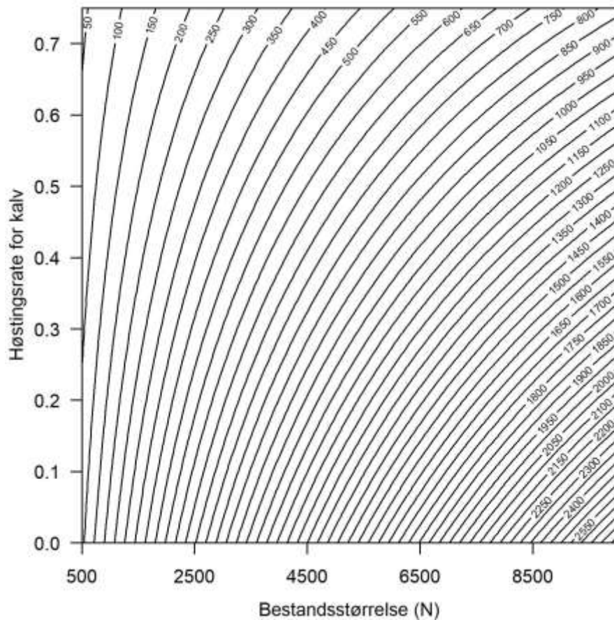
Figur 6: Den effektive bestandsstørrelsen ( N_e ) hos rein for kombinasjoner av total bestandsstørrelse ( N ) og høstingsraten for kalver. Høstingsratene til de andre alders- og kjønnklassene er holdt ved deres gjennomsnitt ( h_{f,1} = 0.078 , h_{f,2} = 0.129 , h_{m,1} = 0.181 , h_{m,2} = 0.156 ), noe som gir vekstrater \lambda = 1.048 , ved h_{f,0} = h_{m,0} = 0 og \lambda = 0.883 ved h_{f,0} = h_{m,0} = 0.75 . Alders- og kjønnsstrukturen til bestanden før jakt er satt lik alders- og kjønnsstrukturen som er estimert for 2021 ( U_{f,0} = 0.125 , U_{f,1} = 0.087 , U_{f,2} = 0.427 , U_{m,0} = 0.125 , U_{m,1} = 0.085 , U_{m,2} = 0.151 ).
