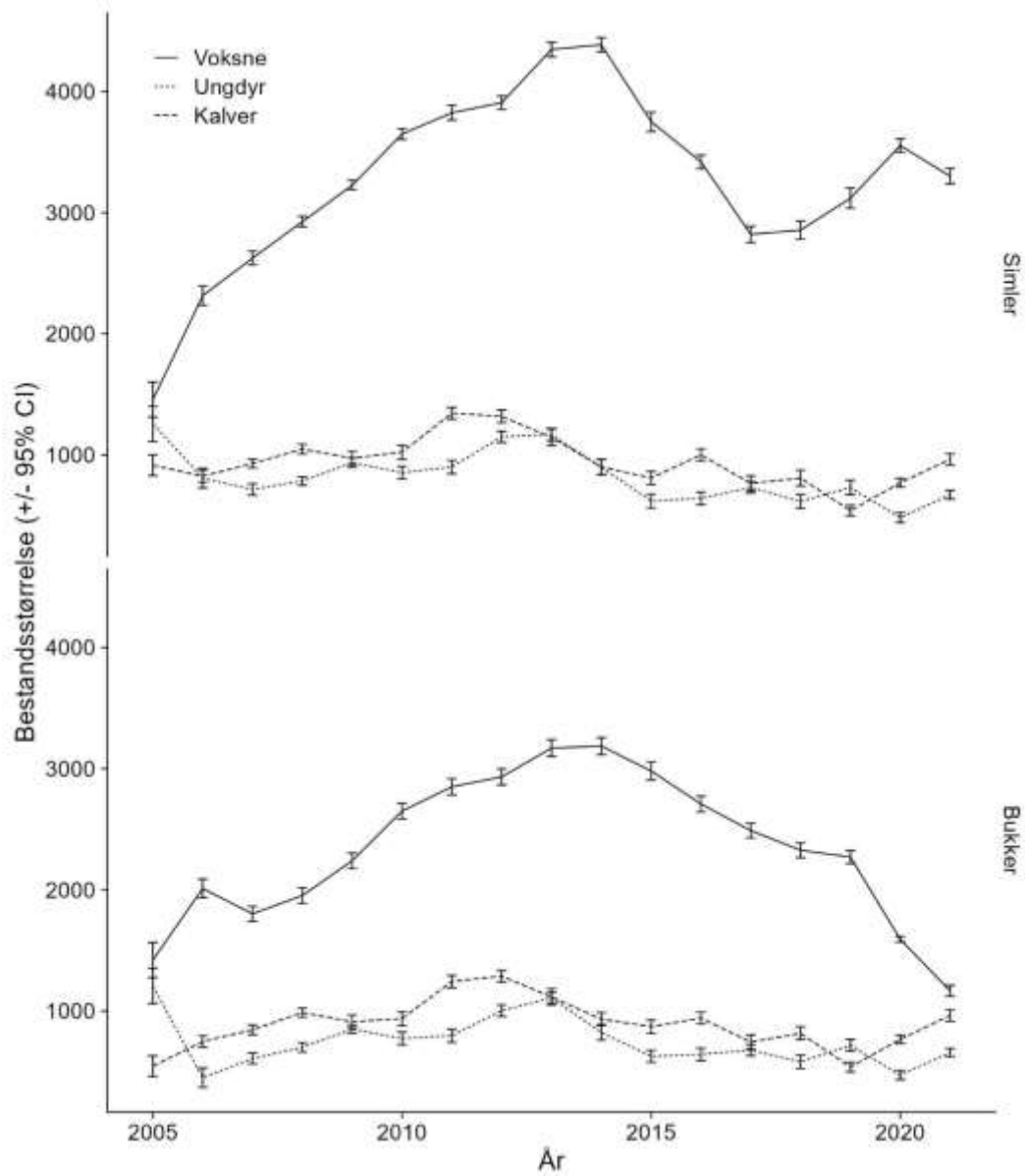
Figur A2: Estimert bestandsstørrelse for hver alders- og kjønnsklasse (gjennomsnitt \pm 95 % konfidensinterval) i reinbestanden på Hardangervidda.
