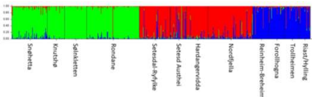
Figur 3 Genetisk struktur for 10 nasjonale villreinområder og fra tamreinbestandene i Trollheimen og Riast-Hylling. Fargene representerer genetiske grupper eller såkalte genetiske signaturer. Illustrasjonen viser at villrein i Rondane-Dovre regionen, villrein i Langfjella-regionen og tamrein har hver sine genetiske signaturer. Den bakenforliggende analysen er gjort på individnivå og viser den genetiske sammensetningen i hvert enkelt individ.
