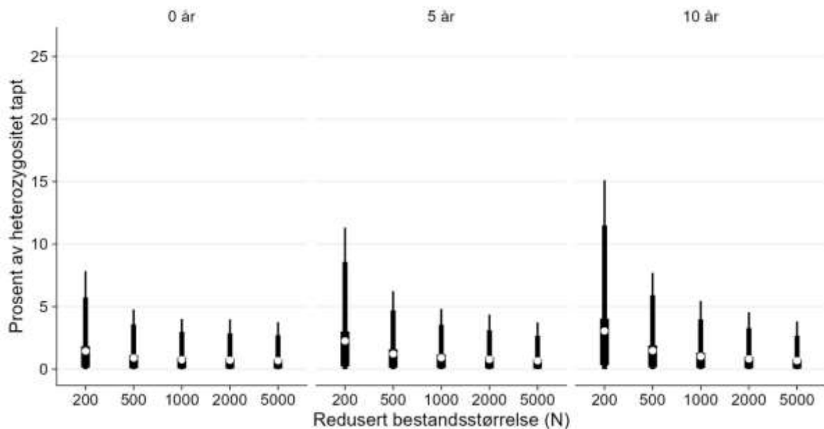
Figur 10: Tap av heterozygositet over 100 år, hvor en starter med bestandsreduksjon som holdes i 0, 5 eller 10 år. 20 % av voksen simle og bukk høstes i perioden med redusert bestand og bestanden holdes stabil ved å skalere høstingsratene til kalv og ungdyr. N_0 = 7725 , p_0 = 0.5 og etter perioden med bestandsreduksjon opphører all høsting slik at bestanden vokser inntil den når N_0 . Ved N_0 holdes bestanden stabil ved å skalere alle de gjennomsnittlige høstingsratene for perioden 2005-2018. Det hvite punktet viser gjennomsnittet, mens 50, 90 og 95 % konfidensintervaller er vist med usikkerhetsstolper av ulik bredde.
