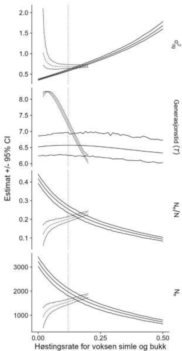
Figur 3: Demografisk varians ( \sigma_{a_g}^2 ), generasjonstid ( T ), forholdet mellom effektiv og faktisk bestandsstørrelse ( N_e/N ) og N_e (gitt N = 7725 i 2021) for ulike høstingsrater for voksen simle og bukk (2.5 år eller eldre). Den heltrukne linjen viser resultatene når høstingsratene for de andre alders- og kjønnklassene holdes ved deres gjennomsnitt ( h_{f,0} = 0.105 , h_{f,1} = 0.078 , h_{m,0} = 0.136 , h_{m,1} = 0.181 ), noe som gir vekstrater \lambda = 1.129 , ved h_{f,2} = h_{m,2} = 0 og \lambda = 0.757 ved h_{f,2} = h_{m,2} = 0.50 . Den stiplede linjen viser resultatene når den gjennomsnittlige høstingsraten til kalver og ungdyr skaleres slik at \lambda = 1 . Ved høstingsrater for voksen simle og bukk mindre enn 2% eller større enn 21% kan ikke \lambda = 1 oppnås. Den prikkete vertikale linjen indikerer parameterverdiene ved den gjennomsnittlige høstingsraten for voksne, (h_{f,2} + h_{m,2})/2 = 0.143 .
