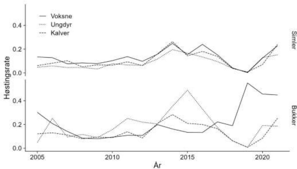
Figur A3: Estimert årlig høstingsrate for hver alders- og kjønnsklasse i reinbestanden på Hardangervidda. Estimaten er basert på rapportert antall dyr som er høstet og den estimerte bestandsstørrelsen til hver alders- og kjønnsklasse.
