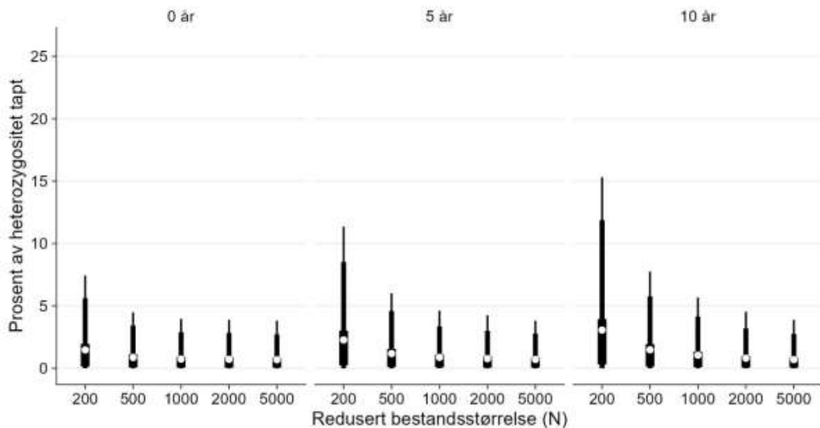
Figur 12: Tap av heterozygositet over 100 år, hvor en starter med bestandsreduksjon som holdes i 0, 5 eller 10 år. Alle høstingsrater skaleres når bestandsstørrelsen holdes stabil. N_0 = 7725 , p_0 = 0.5 og etter perioden med bestandsreduksjon opphører all høsting slik at bestanden vokser inntil den når N_0 og holdes stabil der. Skalerte høstingsrater tar som utgangspunkt de observerte gjennomsnittlige høstingsratene i perioden 2005-2018. Det hvite punktet viser gjennomsnittet, mens 50, 90 og 95 % konfidensintervaller er vist med usikkerhetsstolper av ulik bredde.
