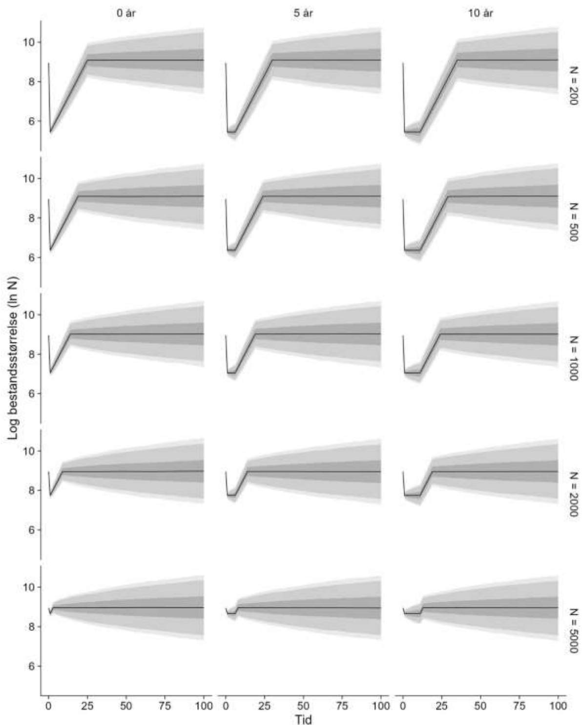
Figur C1: Fordeling av den naturlige logaritmen av bestandsstørrelse over tid i simuleringer hvor en starter med bestandsreduksjon som holdes i 0, 5 eller 10 år og 90 % av voksen bukk høstes mens bestanden holdes stabil ved å skalere høstingsratene til kalv, ungdyr og voksen simle. Skalerte høstingsrater tar som utgangspunkt de observerte gjennomsnittlige høstingsratene i perioden 2005-2018. N_0 = 7725 , \sigma_d^2 = 0.581 og \sigma_e^2 = 0.007 og etter perioden med bestandsreduksjon opphører all høsting slik at bestanden vokser inntil den når N_0 og holdes stabil der. Den heltrukne linjen viser gjennomsnittet og 50, 90 og 95 % konfidensintervaller er vist med de ulike gradene av grått.
