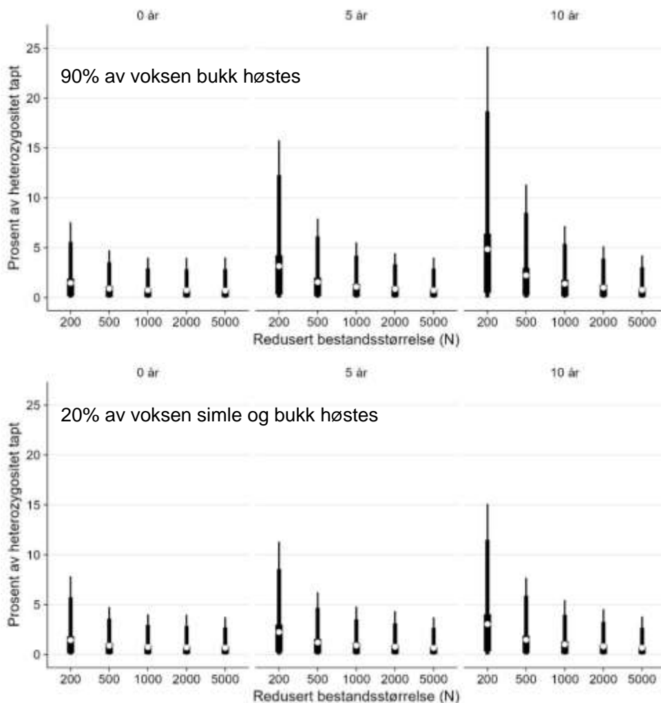
Figur 7 Tap av genetisk variasjon over 100 år, hvor en starter med en bestandsreduksjon som holdes i 0, 5 eller 10 år. 90% av voksen bukk eller 20% av voksen simle og bukk høstes i perioden med redusert bestand, mens bestanden holdes stabil ved å skalere høstingsratene til kalv og ungdyr. Etter perioden med bestandsreduksjon opphører all høsting slik at bestanden vokser inntil den når bestandsstørrelsen før uttaket startet og holdes stabil der med høstingsrater proporsjonale til gjennomsnittene for perioden 2005-2018. Det hvite punktet viser gjennomsnittet av simuleringene, mens 50, 90 og 95% konfidensintervaller er vist med usikkerhetsstolper av ulik bredde.
