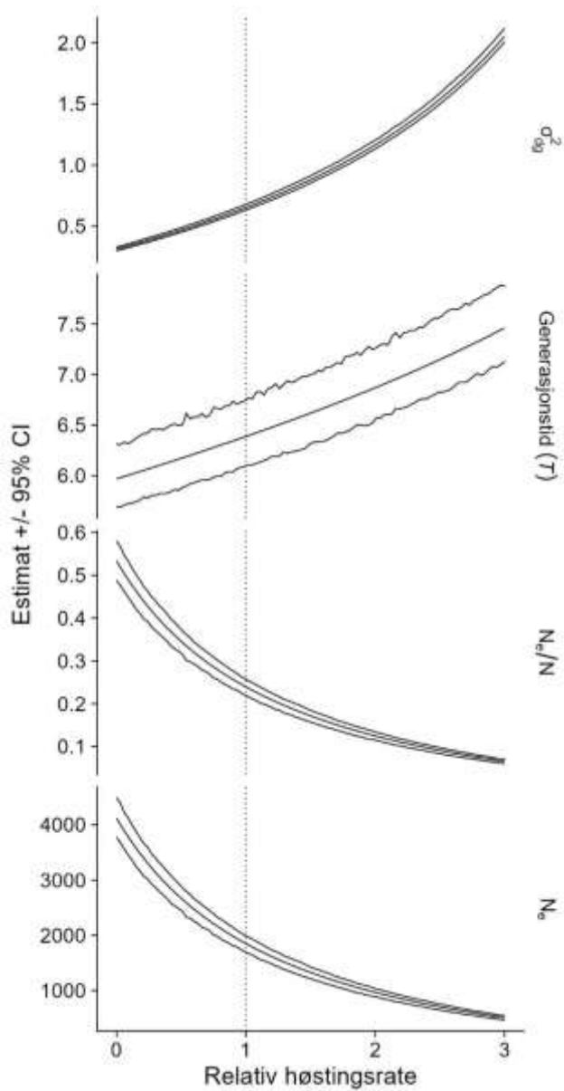
Figur 7: Demografisk varians ( \sigma_{ag}^2 ), generasjonstid ( T ), forholdet mellom effektiv og faktisk bestandsstørrelse ( N_e/N ) og N_e (gitt N = 7725 i 2021) for ulike relative høstingsrater hos rein. Høstingsratene er gitt relativt til gjennomsnittsratene, slik at en relativ høstingsrate på 2 er lik en dobling av de gjennomsnittlige høstingsratene. Vekstraten \lambda = 1.163 når de relative høstingsratene er satt til 0 (ingen høsting) og \lambda = 0.757 når de relative høstingsratene er 3. Den prikkete vertikale linjen indikerer parameterverdiene ved de observerte gjennomsnittlige høstingsratene.
