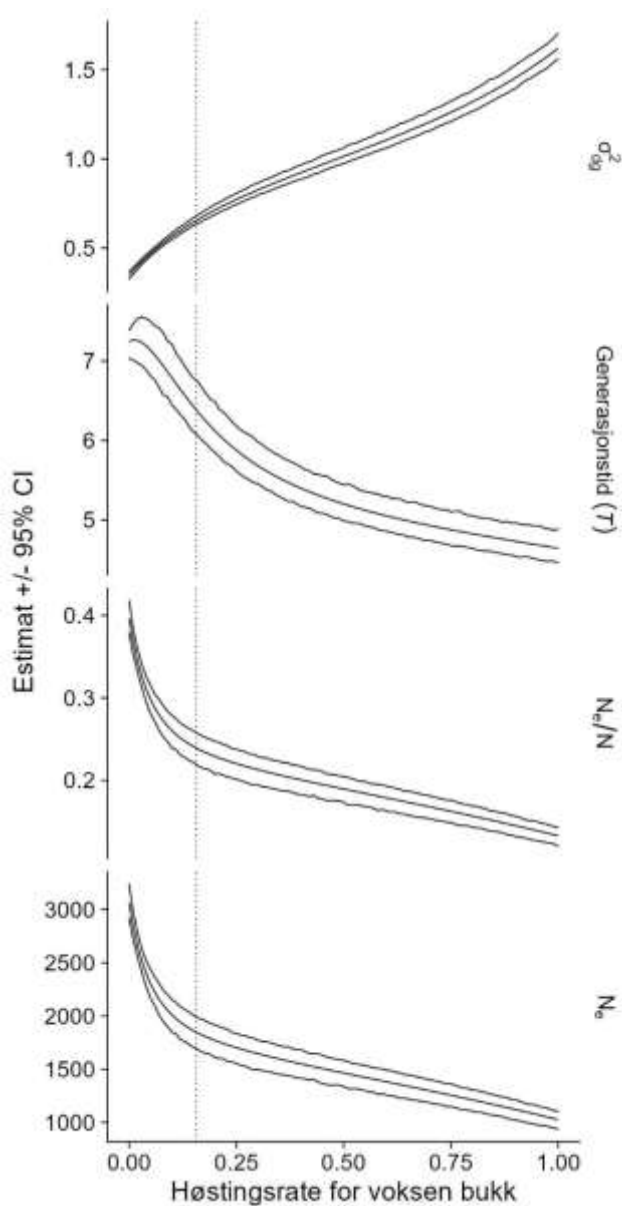
Figur 1: Demografisk varians ( \sigma_{ag}^2 ), generasjonstid (T), forholdet mellom effektiv og faktisk bestandsstørrelse ( N_e/N ) og N_e (gitt N = 7725 i 2021) for ulike høstingsrater for voksen bukk (2.5 år eller eldre). Høstingsratene for de andre alders- og kjønnsklassene holdes ved deres gjennomsnitt ( h_{f,0} = 0.105 , h_{f,1} = 0.078 , h_{f,2} = 0.129 , h_{m,0} = 0.136 , h_{m,1} = 0.181 ), noe
