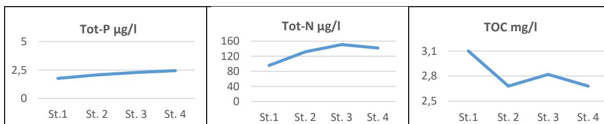
Figur 10. Analyseresultater: Middelverdier for totalt innhold av fosfor, nitrogen og organisk karbon.
