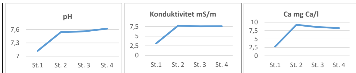
Figur 8. Slettenelva. Analyseresultater: Middelveier for pH, konduktivitet og kalsium.
