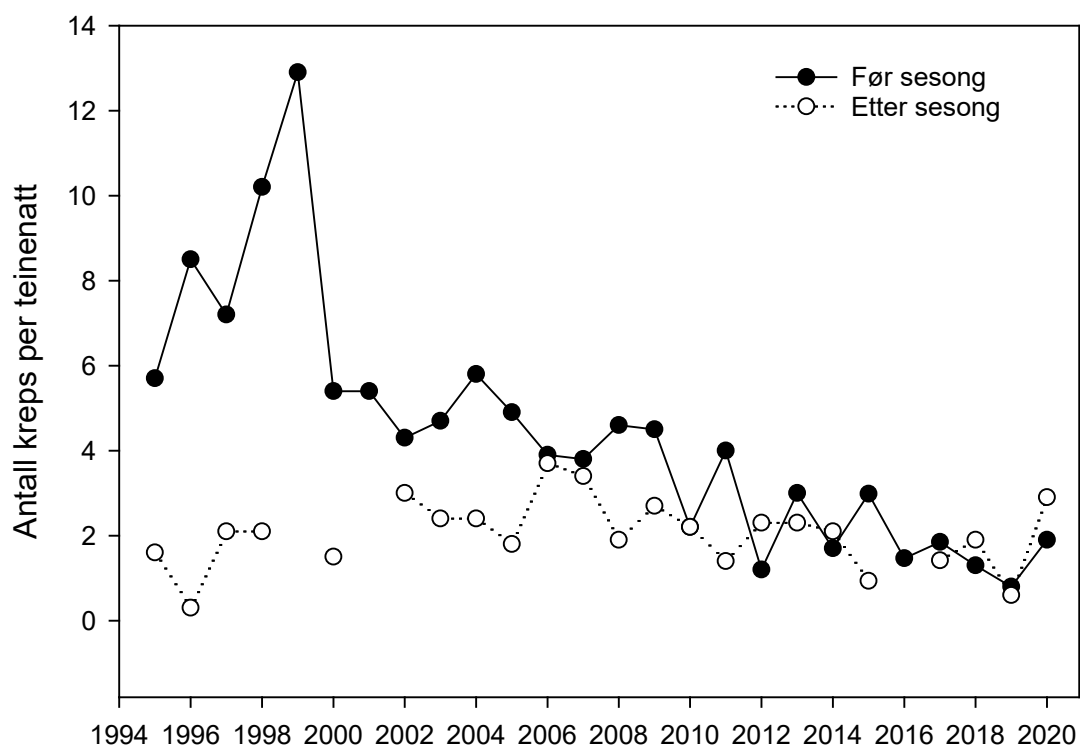
Figur 5.18.3. Antall kreps per teinenatt for prøvefiske før og etter krepseseasonen i Harasjøen for årene 1995-2020.
