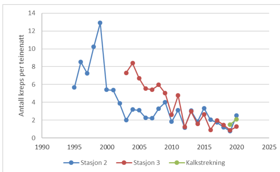
Figur 5.18.4. Utvikling i antall kreps per teinenatt under prøvekrepsing på stasjon 2, stasjon 3 og på den nylig anlagte kalksteinsstrekningen i Harasjøen i årene 1995-2020.
