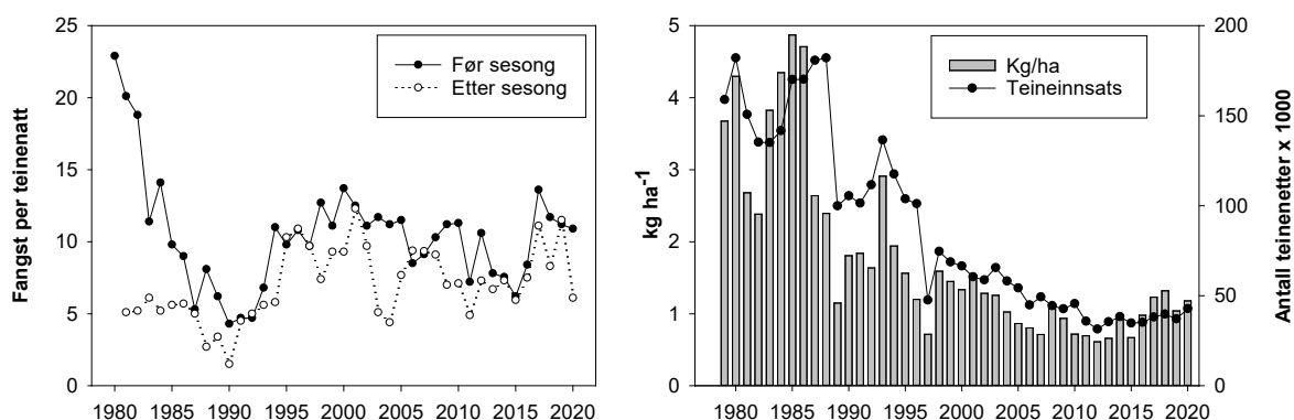
Figur 5.6.2. Grafen til venstre viser utvikling i antall kreps per teinenatt (17.5 mm og 21 mm maskevidde) i Steinsfjorden før og etter sesong i perioden 1981-2020. Grafen til høyre viser utviklingen i fangsttinnssats og totalt uttak av kreps per ha. For eksakte tall, se vedlegg 1 .
