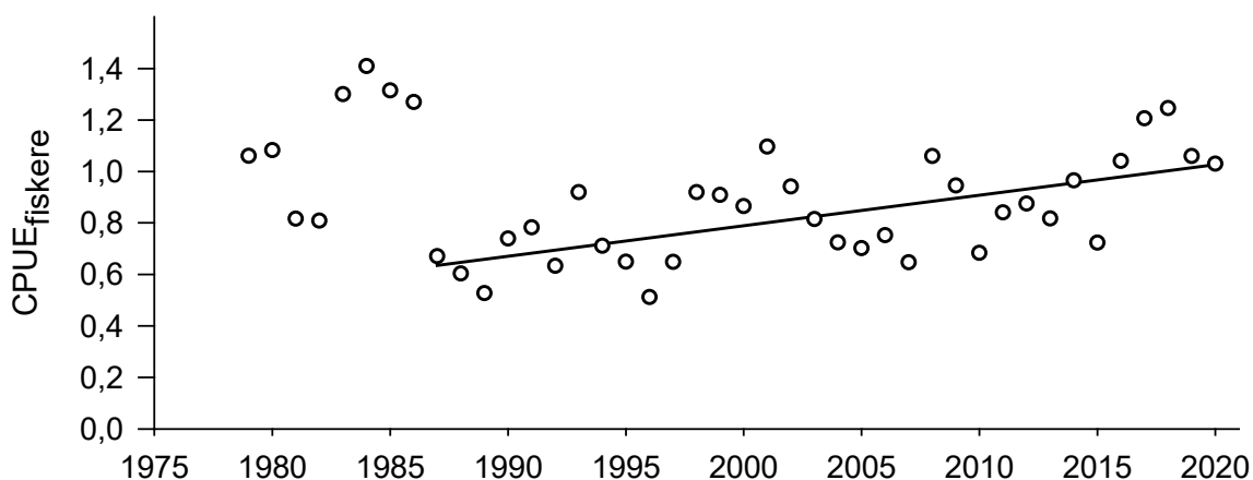
Figur 5.6.3. Utvikling i antall kreps per teinenatt for krepsefiskere i Steinsfjorden i perioden 1979-2020. Trendlinje er lagt for å illustrere utviklingen i fiske etter kollapsen i 1986.
