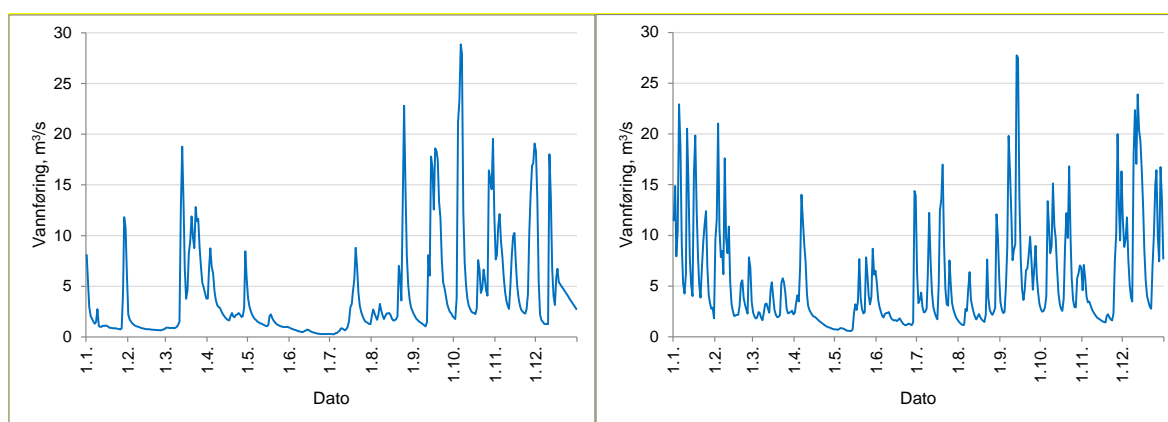
Figur 3. Vannføring i Ogna (døgnmiddel) ved Hetland i 2010 (til venstre) og 2011 (til høyre). Data fra NVE.
