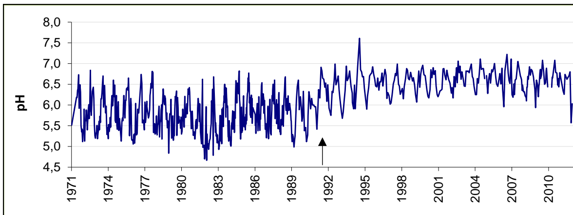
Figur 4. Langtidsserie (1971-2011) for pH på stasjon ovenfor samløp med Hetland kraftverk i Ogna, Rogaland. Pil angir tidspunkt for når permanent kalking av vassdraget kom i gang. Fra Saksgård & Schartau (2012).
